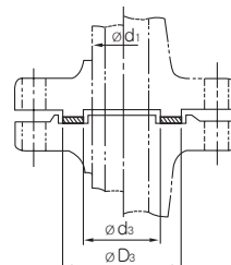
Tongue & Groove Type
